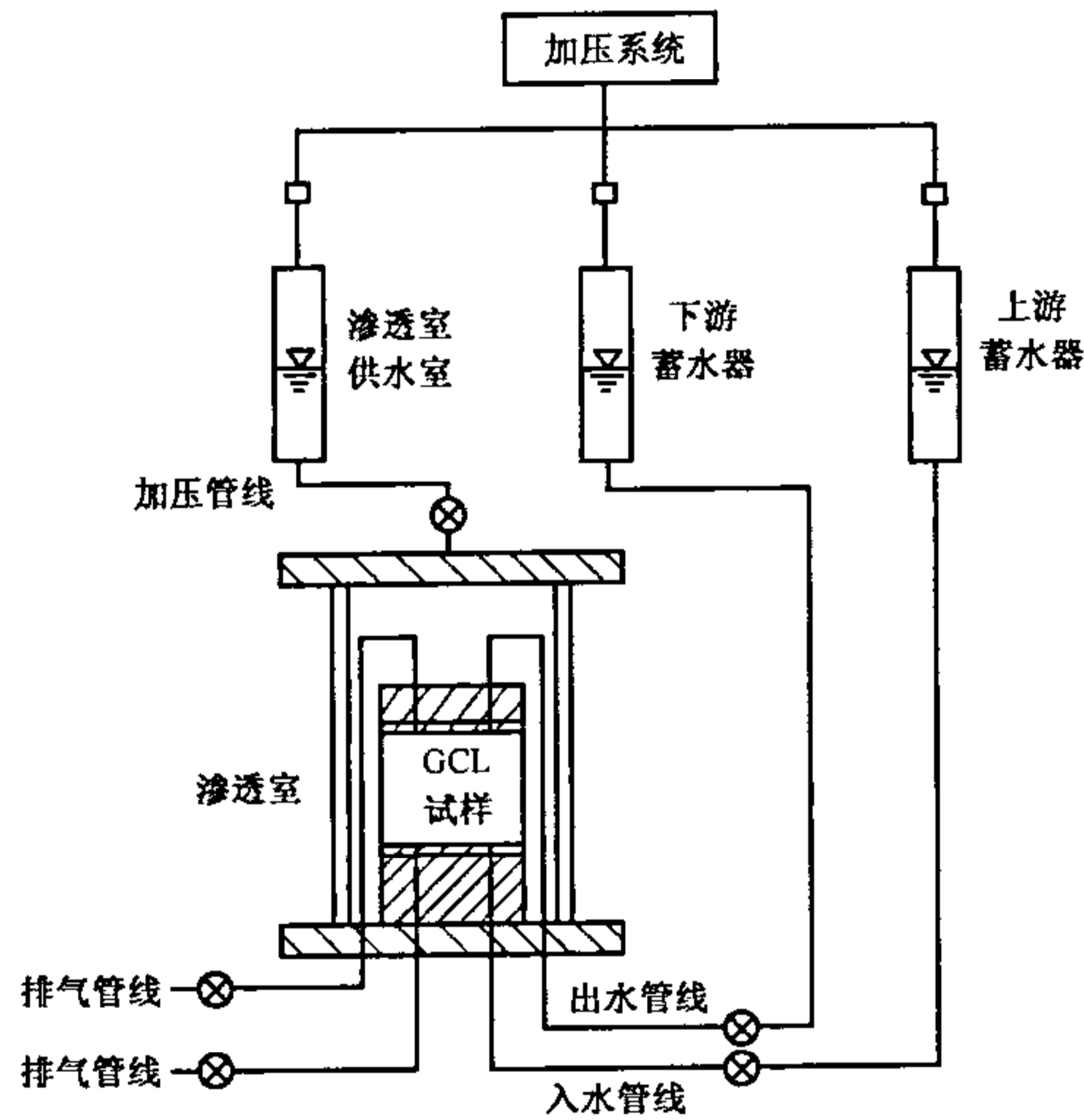
图 A.1 渗透系数测定装置
