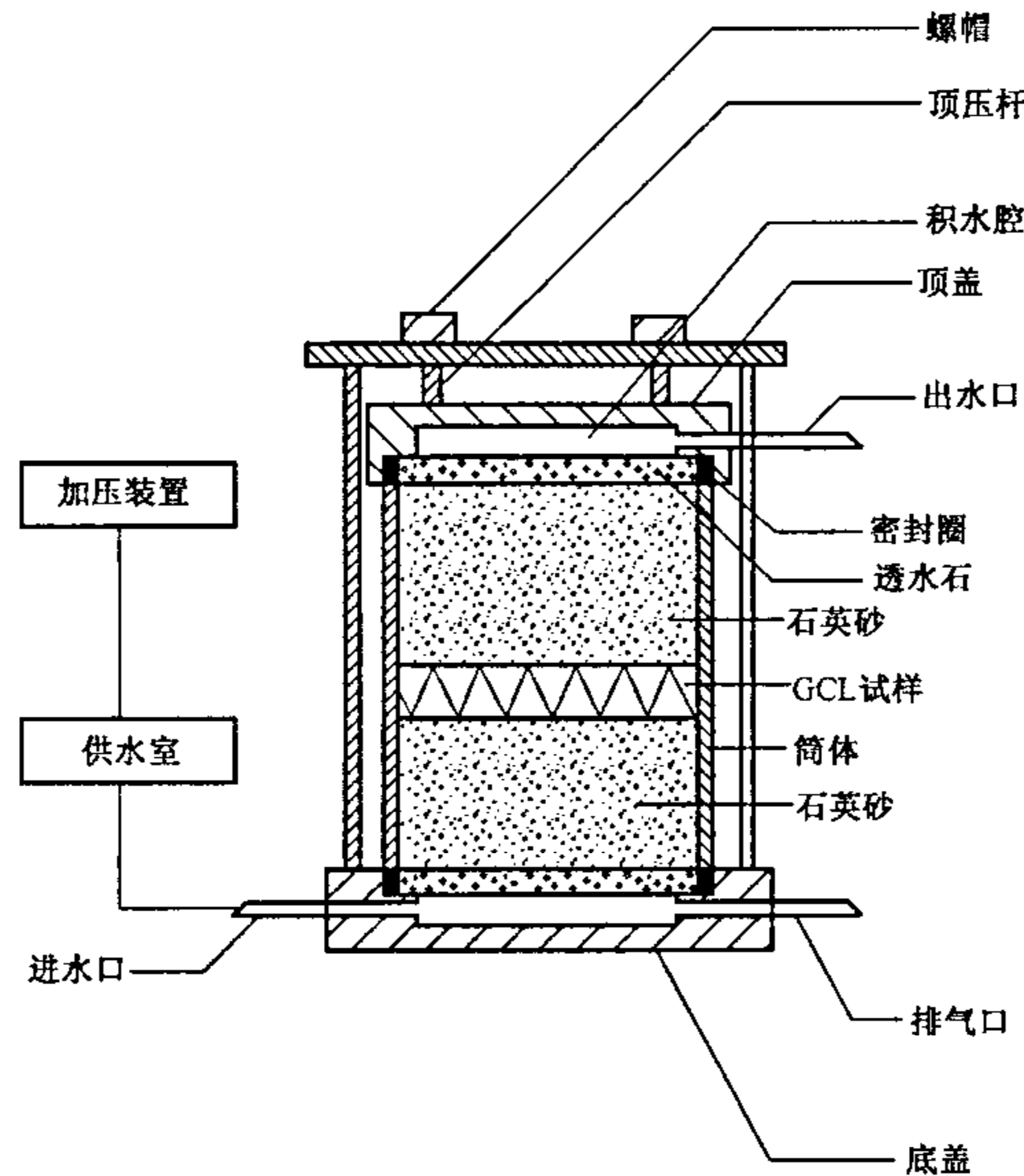
图 B.1 南 55 型渗透仪装置
